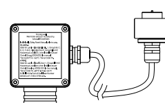
Kit opzionale di montaggio a distanza per sensore XNX EC
